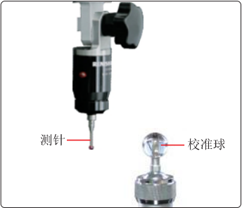
探针(选配), 包含Ø2mm和Ø3mm测针, Ø25mm校准球, 测量精度10µm
